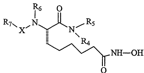
(IIIb)
